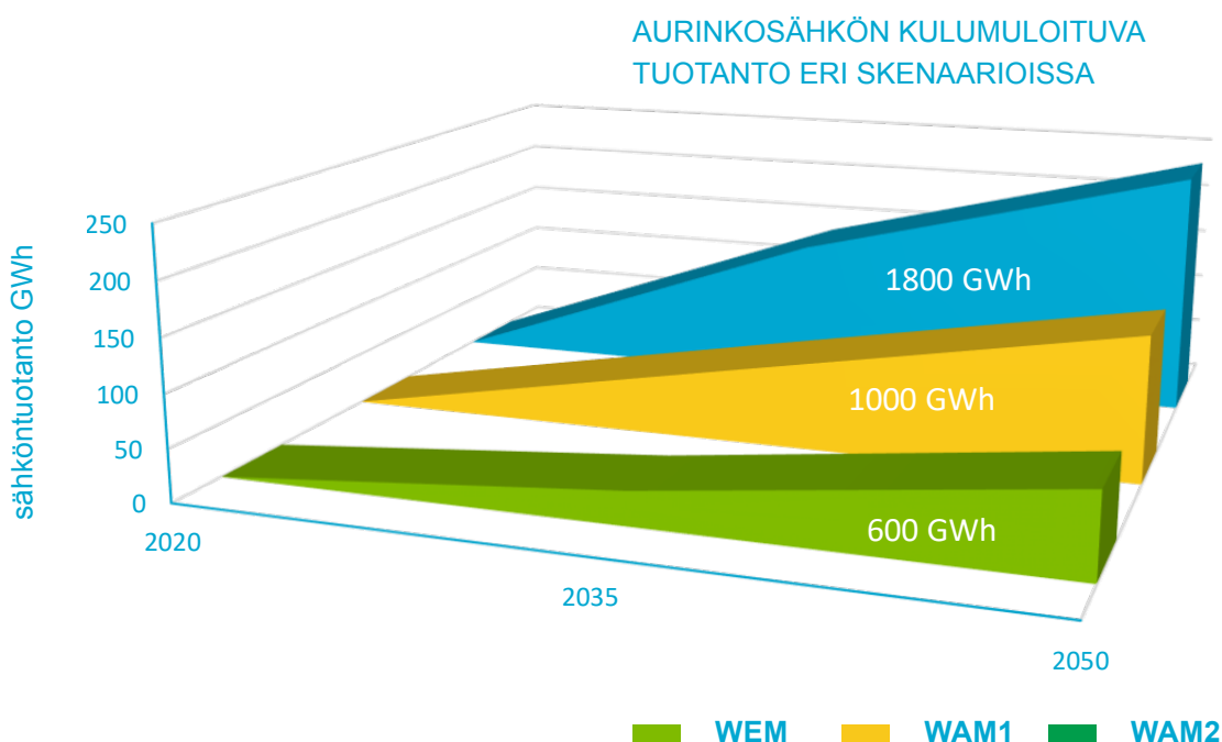
Kuva 6.5.2.1. Tuotetun aurinkosähkön määrä eri skenaarioissa ajan funktiona
