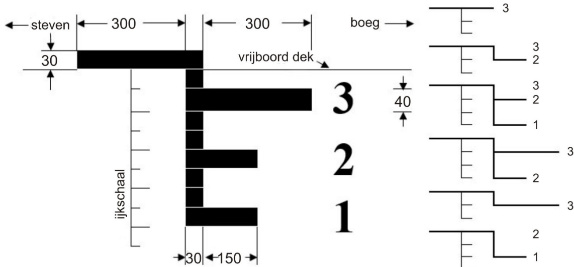
Schets 2
